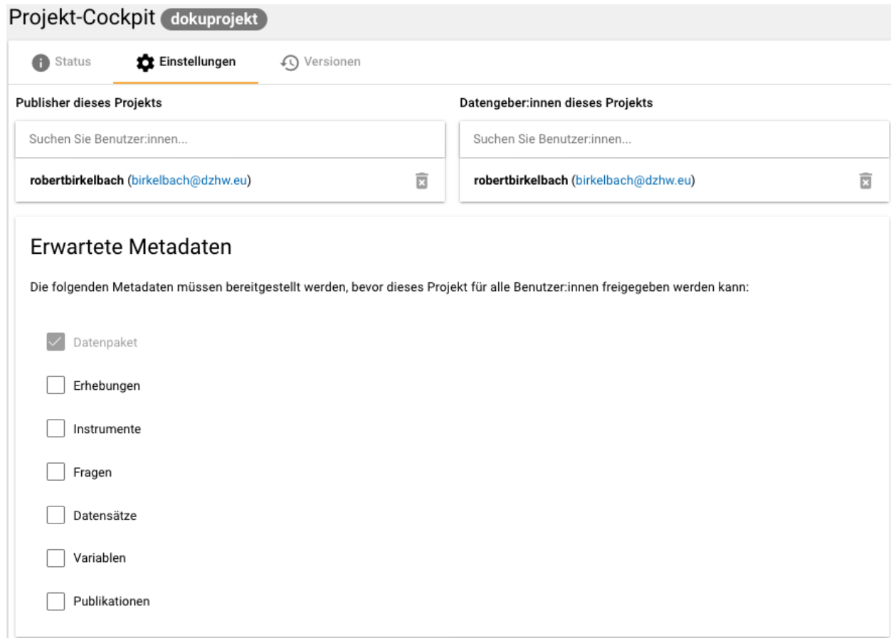
Abb. 3.2: Projekt-Cockpit Einstellungen
